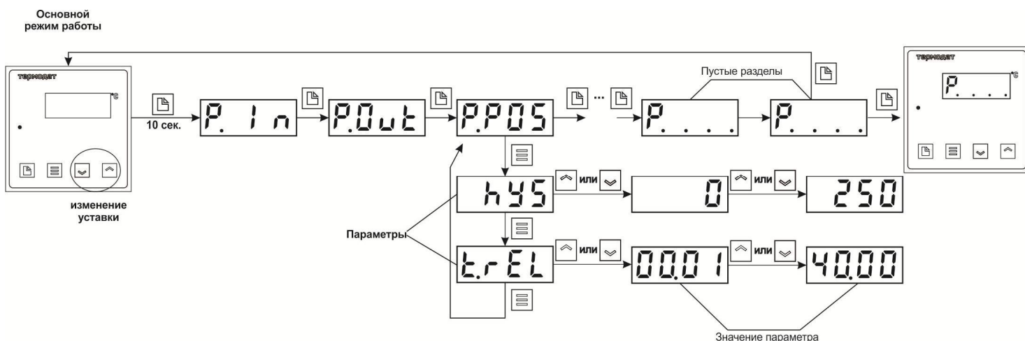
Рисунок 3 – Схема расположения разделов (групп параметров) и параметров в режиме настройки
