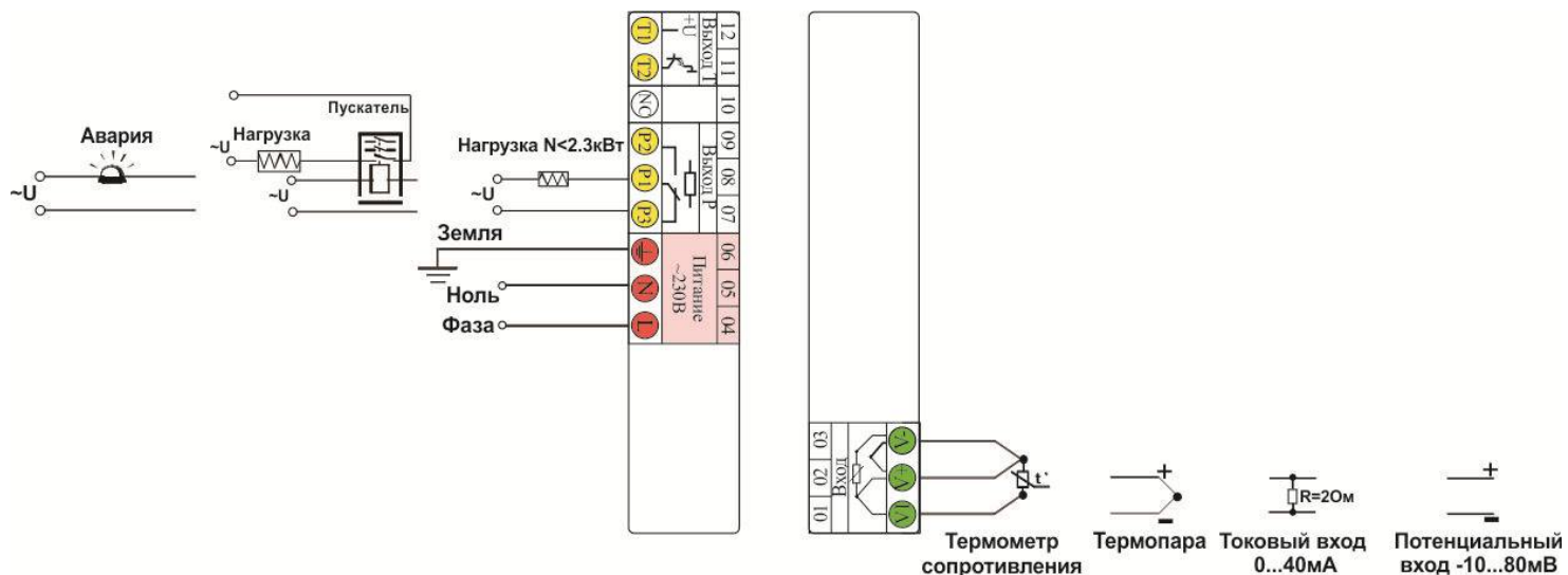
Рисунок 6 – Типовая схема подключения при использовании Т выхода. Для напряжения питания 24В, контакт «N» – «-U», «L» – «+U».
