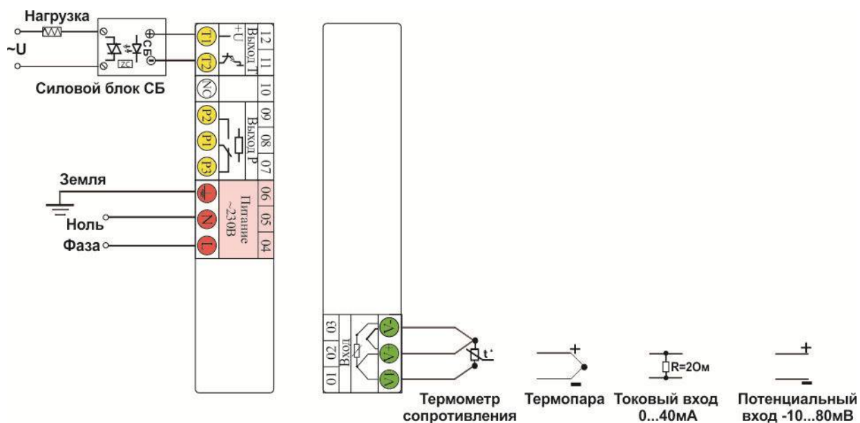
Рисунок 6 – Типовая схема подключения при использовании Т выхода. Для напряжения питания 24В, контакт «N» – «-U», «L» – «+U».
