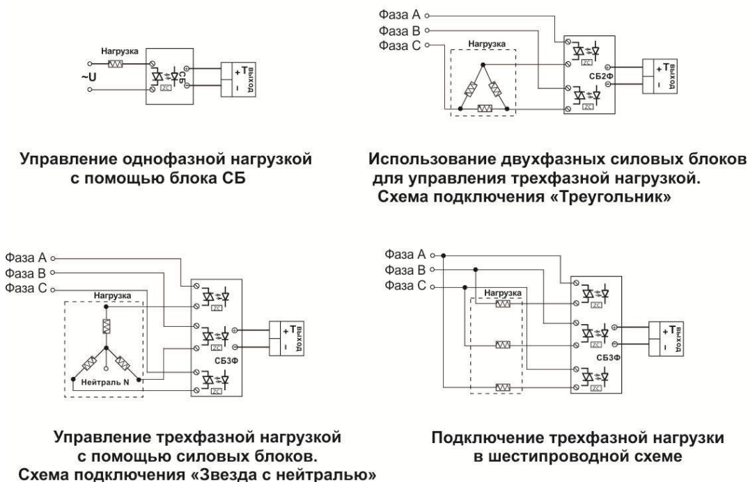
Рисунок 5 – Схемы подключения транзисторного выхода
