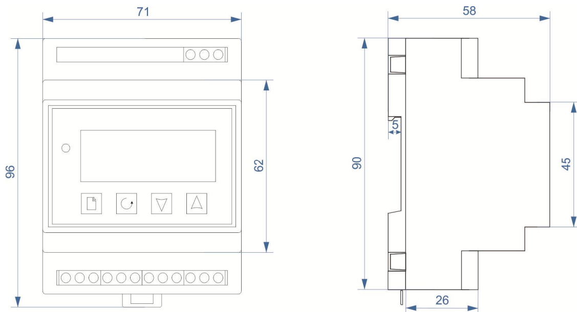
Рисунок 8 – Габаритные размеры прибора 10M7-P4/Б
